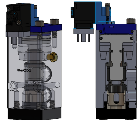
УЛУЧШЕННЫЙ ВАРИАНТ С ПОРШНЕМ
