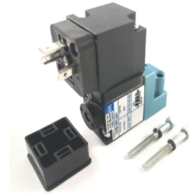
ПИЛОТНЫЙ КЛАПАН ОБРАЗЦА СЕРИИ UNIVERSAL, ПР-ВО MAC
